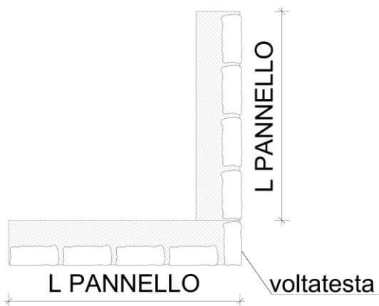
Figura 1 - esempio in di voltatesta d'angolo tra pannelli
