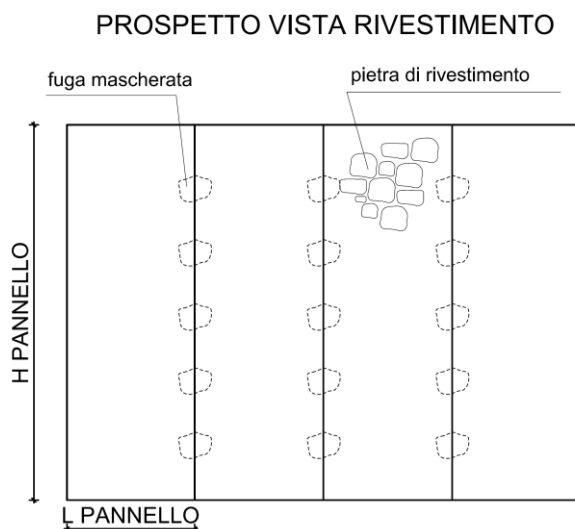
Figura 1 - esempio tipo di prospetto con individuazione del passo della fuga mascherata su lastra rivestita
